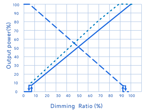
输出功率Vs.调光信号
